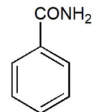
benzamida
