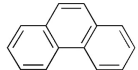
fenantreno
