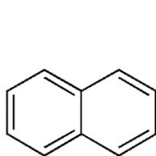
naftaleno
