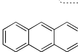
antraceno
