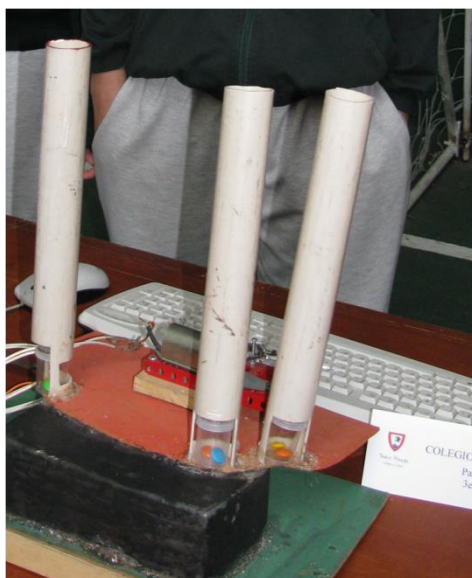
Figura 7: Dispensador robotizado de medicación para personas con Alzheimer
