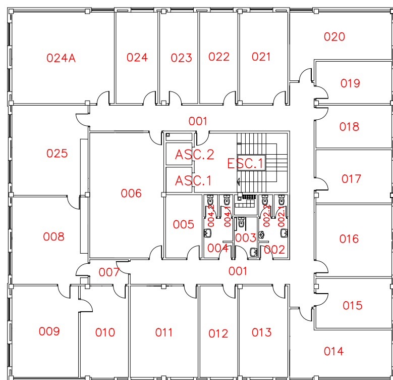
PLANTA CUARTA
