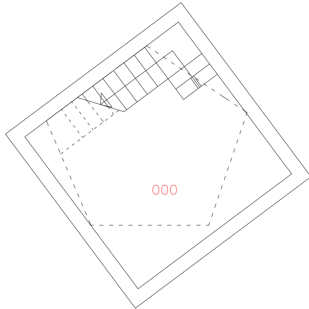
PLANTA SOTANO
