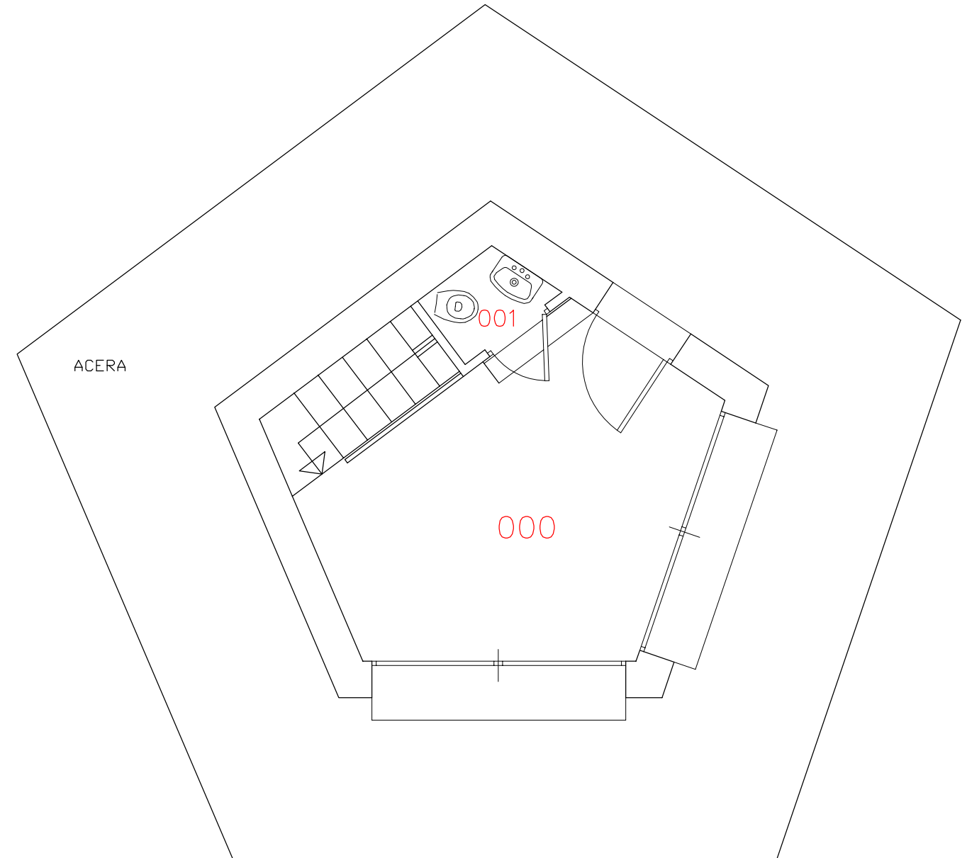
PLANTA GENERAL
