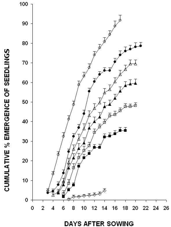
Figura 1. Emergencia acumulada de semillas de Suaeda nudiflora en respuesta a la salinidad del suelo. 0.3 \text{ dSm}^{-1} (○), 3.9 \text{ dSm}^{-1} (●), 6.0 \text{ dSm}^{-1} (△), 7.9 \text{ dSm}^{-1} (▲), 10.0 \text{ dSm}^{-1} (□), 12.1 \text{ dSm}^{-1} (■) and 13.9 \text{ dSm}^{-1} (◇). Las barras de error representan ES.
