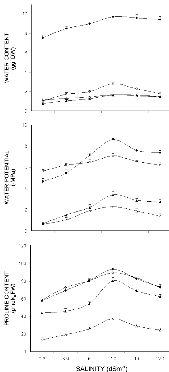
Figura 2. Efecto de la salinidad del suelo en: A. contenido de agua (gg -1 DW); B. potencial hídrico (-MPa); C. contenido de prolina (μmol/g FW) de hojas (●), tallos (○), raíces primarias (▲) y secundarias (Δ) de Suaeda nudiflora . Las barras de error representan SE.
